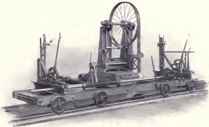
Fig. 34. Band-Saw.
