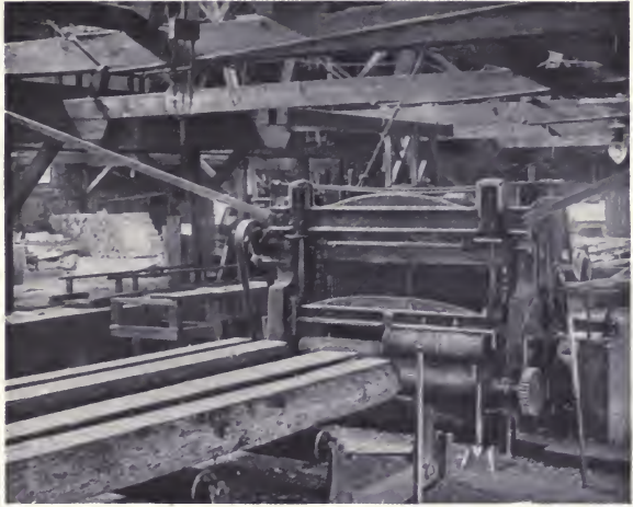
Fig. 33. Gang-Saw.
