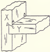
28 Dovetail dado
