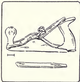
Fig. 110. Scrub-Plane.
