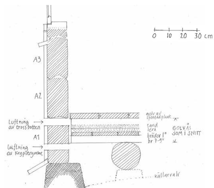
Snitt 5-5 genom A-väggen där trossbotten är luftad.
