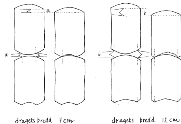
Figur 2.11. Med ett verktyg (timmerdrag, dragjärn m fl beteckningar) förs den undre stockens form över till den övre stocken. Avståndet a och b mellan verktygets skänklar påverkar dragets bredd. Omvänt kan man också säga att dragets bredd ("hur mycket man drar stocken") påverkar hur mycket varje vägstock sjunker. De breda dragen ser man vanligen i vältimrade hus som ska vara varma där draget ger möjlighet till ordentlig drevning. Illustration: Anna Blomberg.
