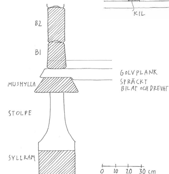
Snitt A-A
