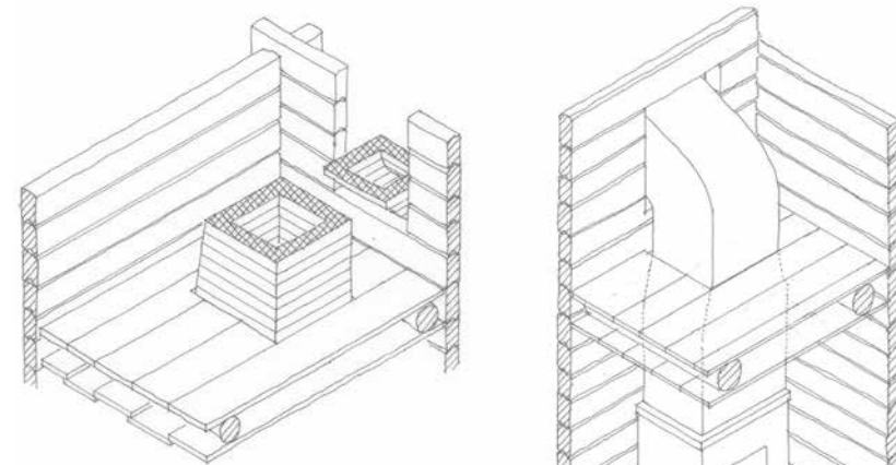
Perspektiv av eldstaden i kammaren och hur den ansluter till skorstenspipan på vinden.
