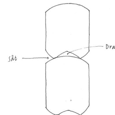
Figur 2.9. Draget är den ränna på stockens undersida som huggs ut för att väggen ska bli tät genom att ”trä tar i trä”. Sät är benämningen på mötet mellan över- och understock på dragets utsidor. Illustration: Anna Blomberg.
