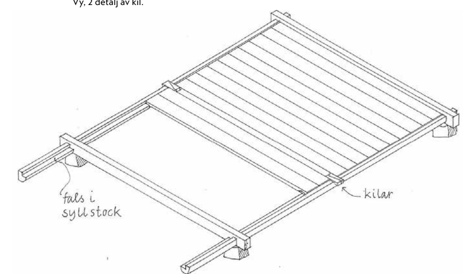
Syllvarvet utlagt och golvplankorna med kilar läggs in Samtliga illustrationer: Anna Blomberg.
