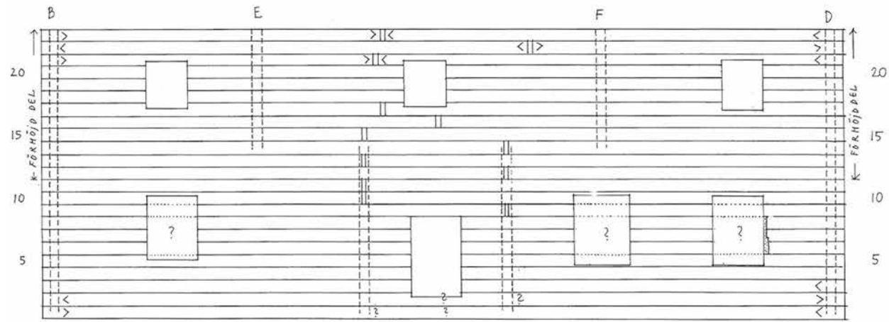
VÄGG A
