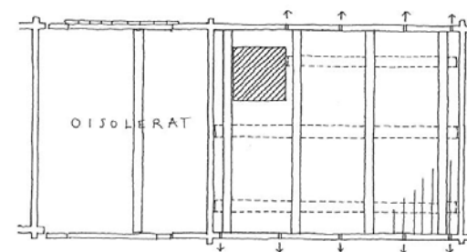
Plan över bottenbjälklag
