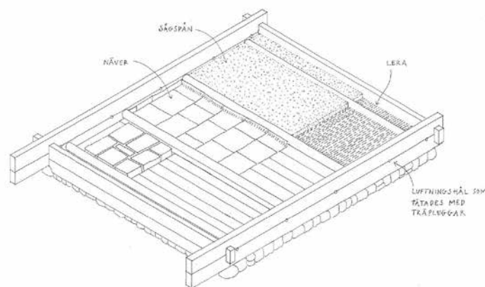
Golvåsarna är intimerade och trossbottenbrädorna ligger på bärlinorna. Samtliga illustrationer av enrumstugan: Kristina Linscott.
