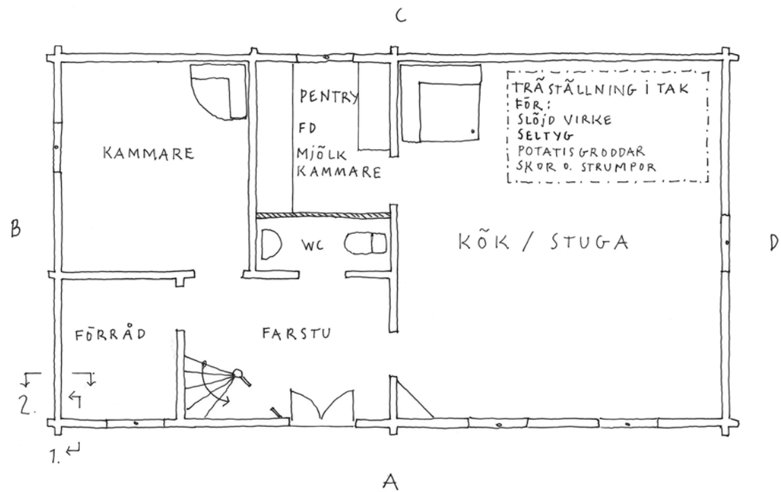
PLAN 1:100
