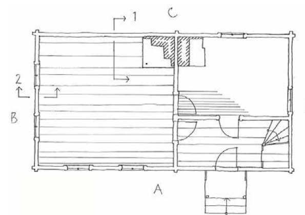
Golvplan
