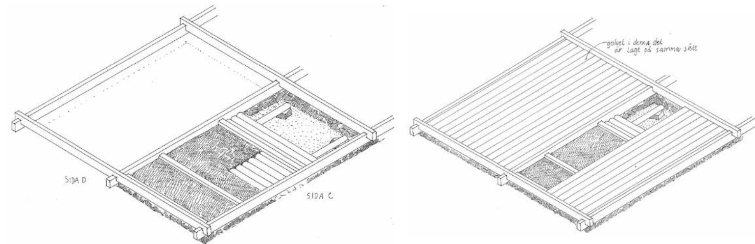
Golvåsar är lagda på trossbotten. Isolering är lagd på mellan golvåsarna.
