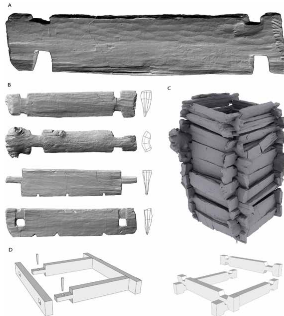
Figur 1.3. Brunnen ifrån Altscherbitz nära Leipzig grävdes fram i samband med exploatering i slutet av 1990-talet. Den lyftes upp i ett block tillsammans med omgivande jordmassor och undersöktes i ett laboratorium. Sex dendrokronologiska prover i konstruktionens ektimmer daterades till 5117-5099 f Kr. Troligtvis en av de äldsta och mest välbevarade timmerkonstruktionerna som är kända.
