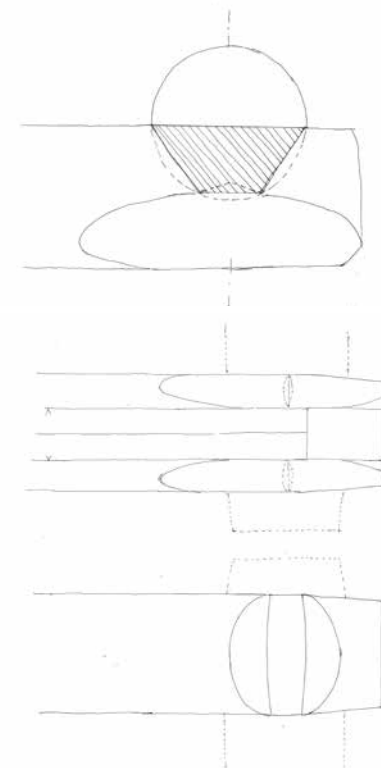
Figur 7.22. Snitt genom knuten och en timmerstock sedd under- respektive ovanifrån av den knuttyp som representerar timmertradition från Dalarna. Illustration: Anna Blomberg
