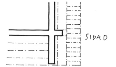
PLAN UTSNITT 1:50 TAKFOT/GAVELSPRÅNG VID HÖRN
