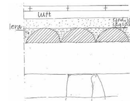
Snitt 4-4 genom golvkol mot D-väggen.
