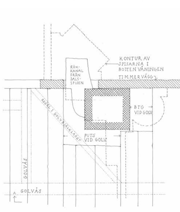
VINDSPLAN SKISS 1:200
