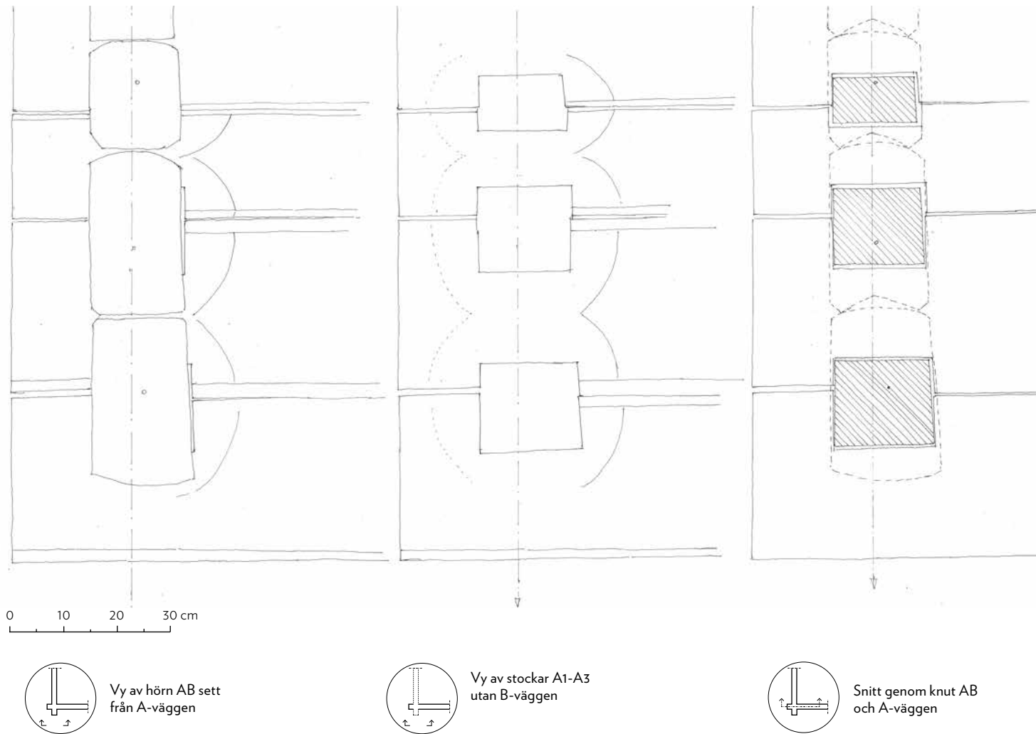
Figur 7.8. Uppmåtningsritning av knuten med: 1. Vy/elevation mot hörn. 2. Samma som 1 men utan tvärgående stockar. 3. Snitt mitt genom väggen, skrafferad yta är knutarna i tvärliggande stockar.
