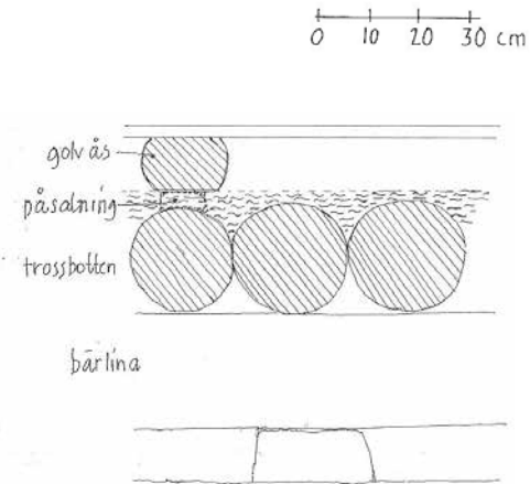
Snitt 2-2 genom golvås och trossbotten av rundvirke
