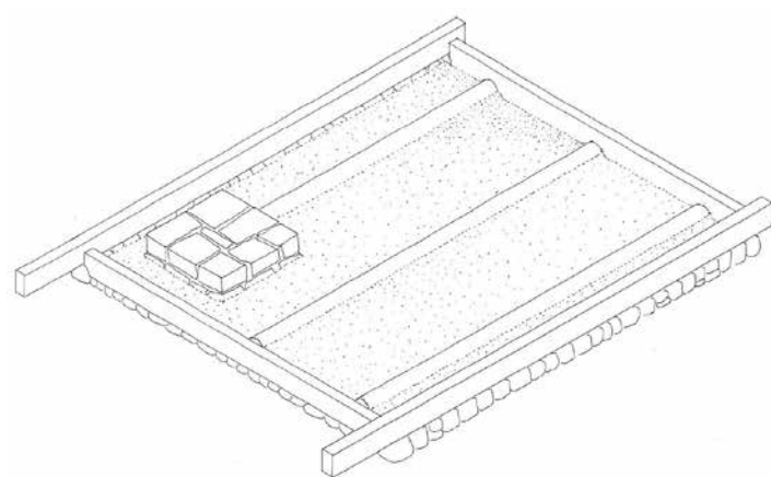
Friliggande bärlinor ligger på upplag av stenar.
