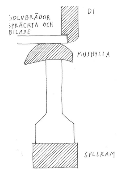
Snitt 1-1
