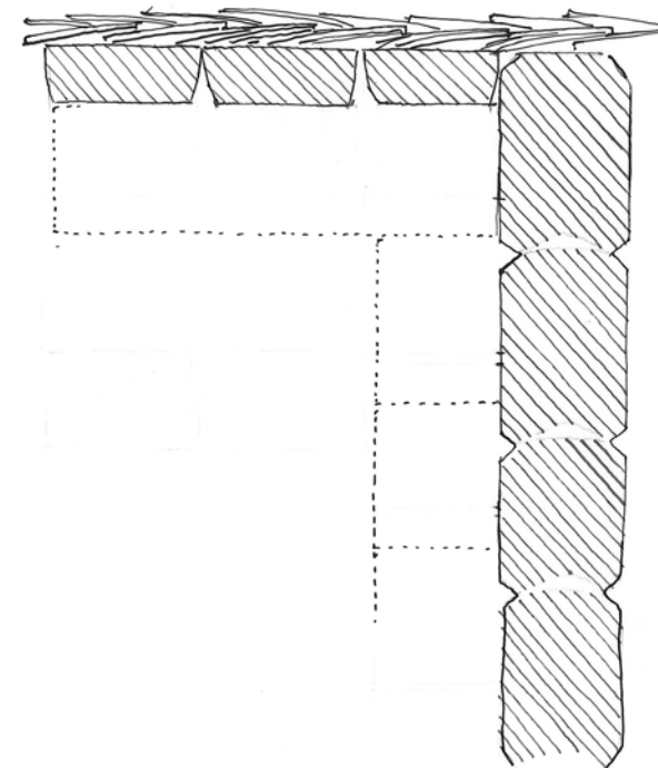
2 GAVELSPRÅNG 1:10
