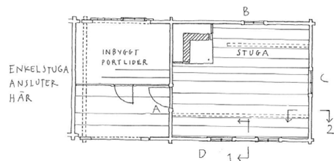
Golvplan
