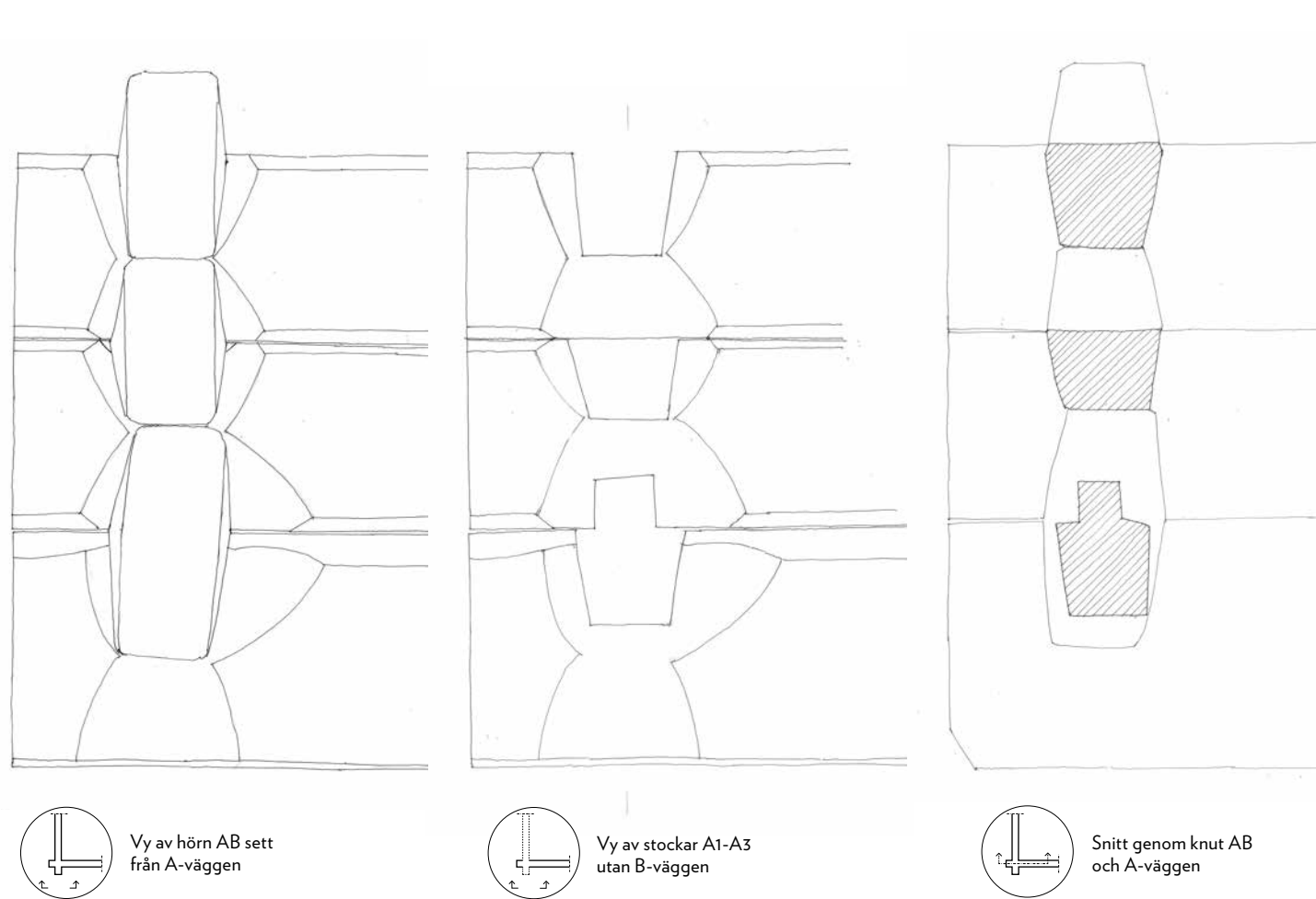
Figur 7.13. Uppmättningsritning av knuten med:
