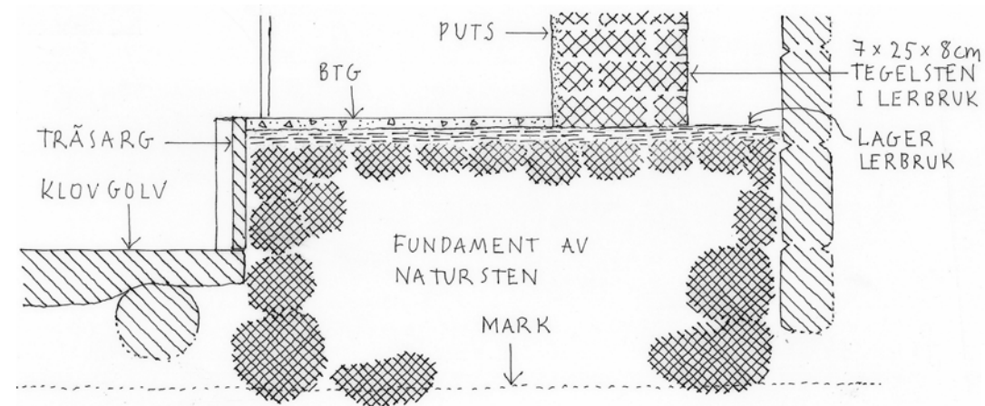
Snitt B-B genom eldstaden i salen.
