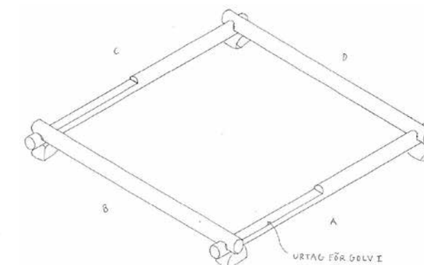
Syllvarvet utlagt på grundstenar Samtliga illustrationer: Anna Blomberg.
