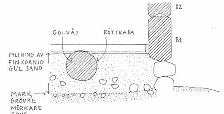
Snitt E-E genom gavelsida B i kammaren.
