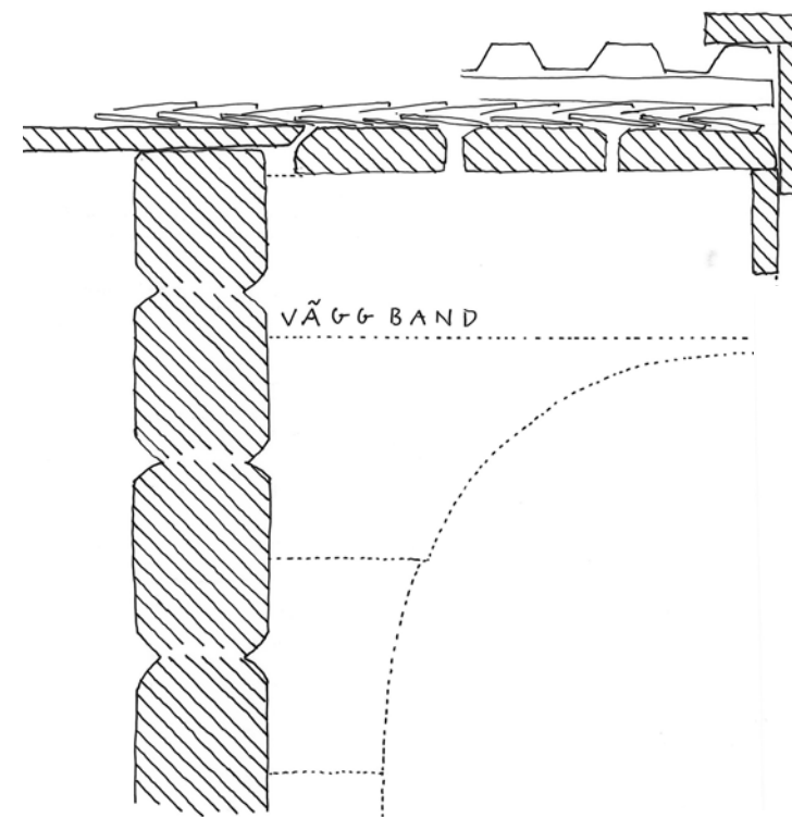
2 GAVELSPRÅNG
