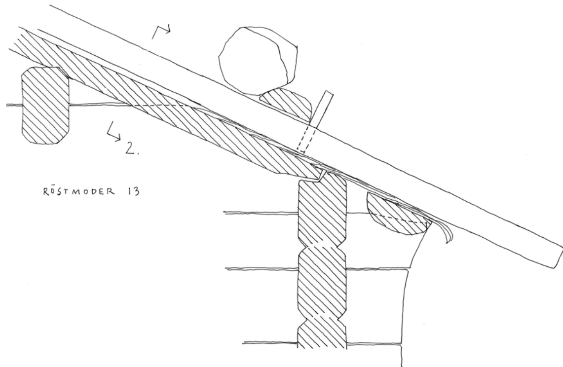
1. TAKFOT 1:10
