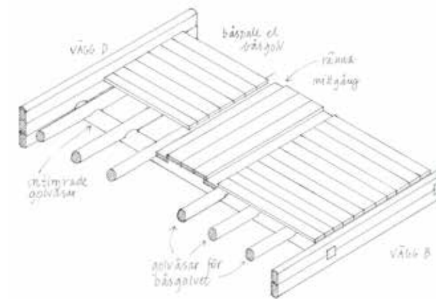
Figur 4.10. Backvallen Ovanåker. Intimrat och tätt men oisolerat golv i ladugården. Illustration: Kristina Linscott.
