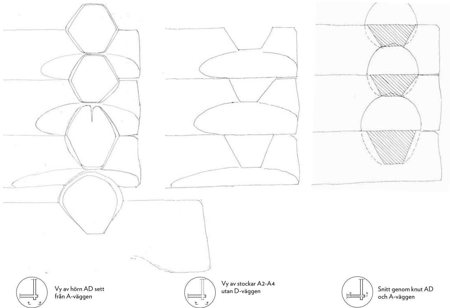
Figur 7.25. Uppmättningsritning av knuten med: 1. Vy/elevation mot hörn. 2. samma som 1 men utan tvärgående stockar. 3. Snitt mitt genom väggen, skrafferad yta är knutarna i tvärliggande stockar.
