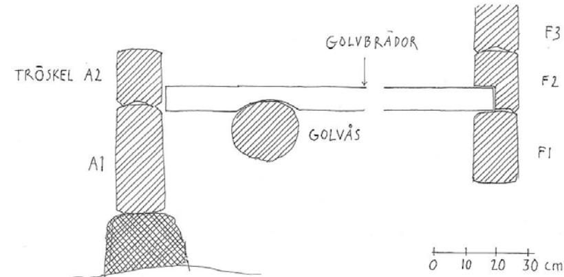
Golvet i farstun, sektion 9-9 och 10-10 Samtliga illustrationer: Anna Blomberg.
