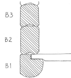
Figur 4.7. Fågelsjö gammelgård. Intimrade golvplankor kan ligga på falsar i syllstocken så att de inte är synliga från utsidan. Illustration: Anna Blomberg.
