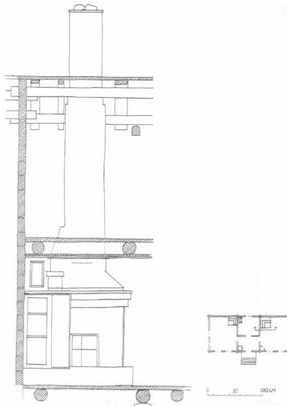
Elevation av kökets eldstad.
