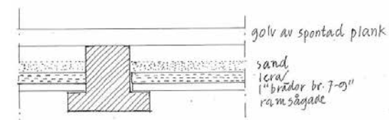
Snitt 1-1 genom golvås och trossbotten. Samtliga illustrationer på uppslaget: Anna Blomberg.
