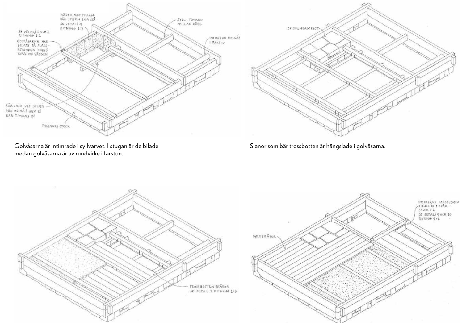
Både trossbottenbräda och sågspånsyllning ligger mellan golvåsarna.
