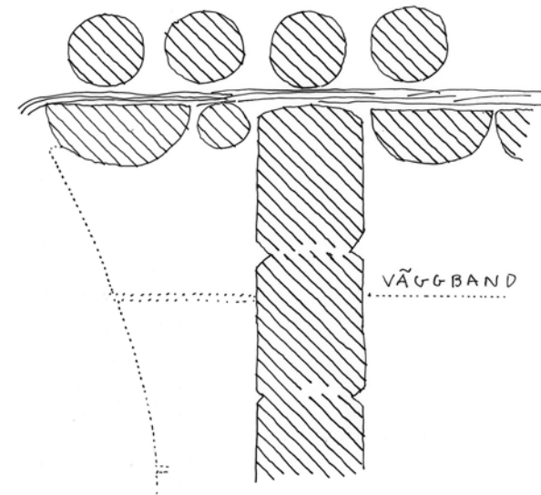
2 GAVEL SPRÅNG 1:10
