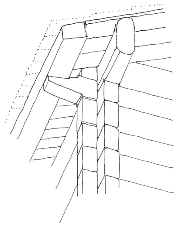
PERSPEKTIV HÖRN
