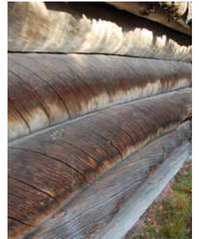
Figur 2.4. Extremt växtvriden ytterved i ett småfåhus som tillhört en fåbod i Älvdalen. Man hade traditionellt kunskap om att den här typen av virke var mycket rötbeständigt och det går att se i många fler byggnader att det används i bottenvarven på fåhus, i syllramar och mushyllor under härbren. Jon Godal benämner detta ”aldersved” (Godal 2012).
