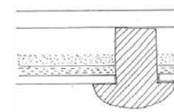
Snitt 2-2 genom golvås och trossbotten.
