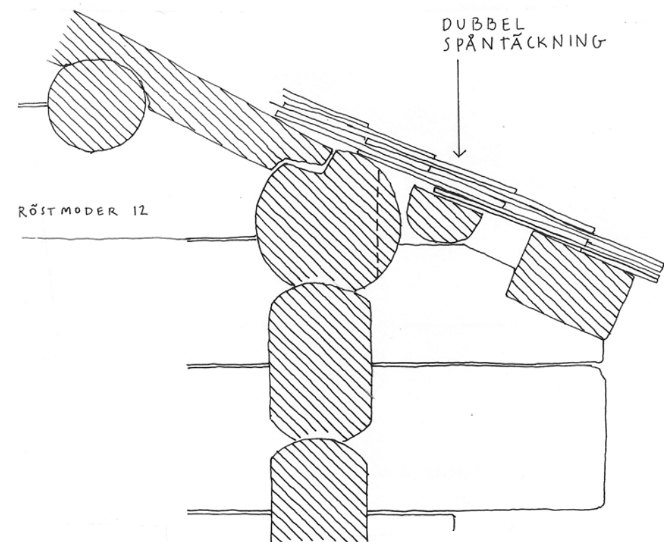
1. TAKFOT 1:10
