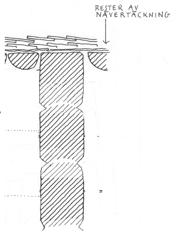
2. GAVELSPRÅNG 1:10
