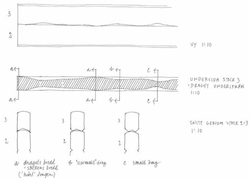
Figur 2.15. En viktig förutsättning för enkel och rationell timring är att använda raka stockar. Om timret trots det har ojämnheter kan möjligheten till att få ett jämbrett drag och likformiga såtar (av funktionella eller estetiska skäl) bero på den tid och kraft man har lagt ner på att bearbeta stockarna ytterligare med yxa och bandkniv. Figuren visar hur dragets bredd varierar om virket har kvar ojämnheter i form av till exempel krökar, kvistbular och "rotslängar". Illustration: Anna Blomberg.
