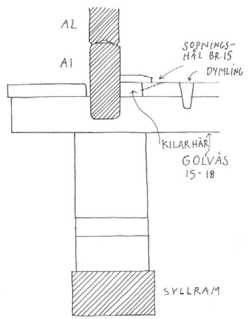
Snitt 2-2
