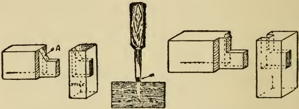
Fig. 127. Haunched Tenon.
