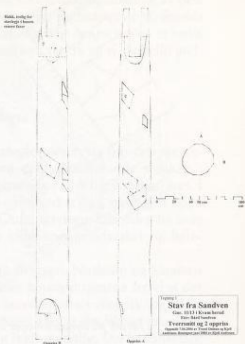
Oppmåling av stav frå Sandven i Kvam
