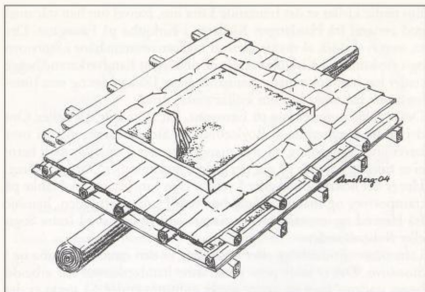
Skisse som viser snitt gjennom bjelkelaga slik vi tenkjer dei var under åren. Den store berebjelken, nedre bjelkelaget og bordlaget oppå det er alt synleg nedanfrå, resten er tenkt. Truleg var det fylt med leire el. l. under åren.
