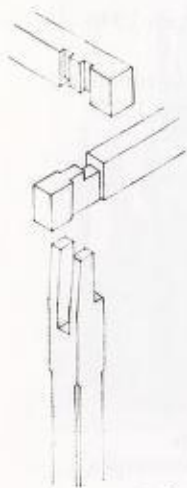
Delar av stav, bete og stavlegje før samanføying.
