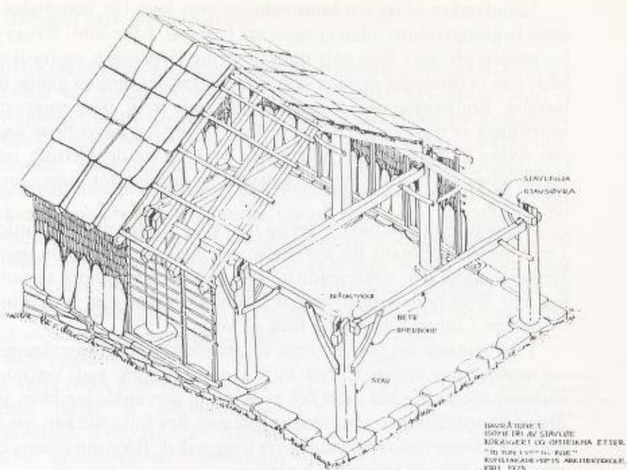
Isometrisk teikning av grindløe frå Havrå på Osterøy teikning ved Kunstakademiets arkitektskole, retta av Nils Georg Brekke.
