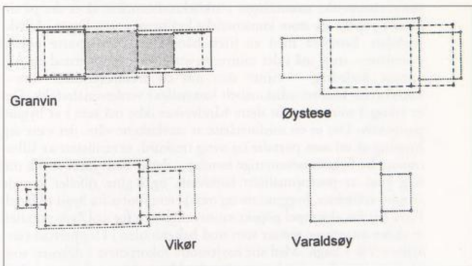
Stavkirker i Hardanger. Grunnplaner. (Fra Lidén 1997).
