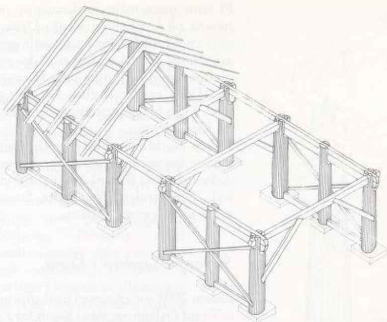
Forsøk på isometrisk snitt av stavløe på Norheim i Kvam
