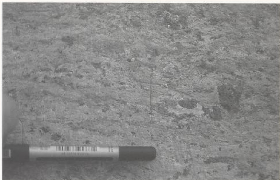
Nærbilde av hjørnestein av kleber i skipet til Kinsarvik kirke. Legg merke til de karakteristiske linsene av magnesitt (fargen er gulbrun) – som forteller at steinen ikke er fra Kvitmo.
