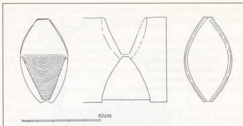
Detalj av hovhogg i Storstovo, frå sørvestre hjørne, snitt gjennom halsen t.v. Form, plassering, kinning i overhogget o.m. er likeins begge stader. Stokkane er grovve enn dei som er utførde. Dei utførde fekk ikkje profilerte novendar som dei på Aga. (Frå bd. V s. 179 ø)
