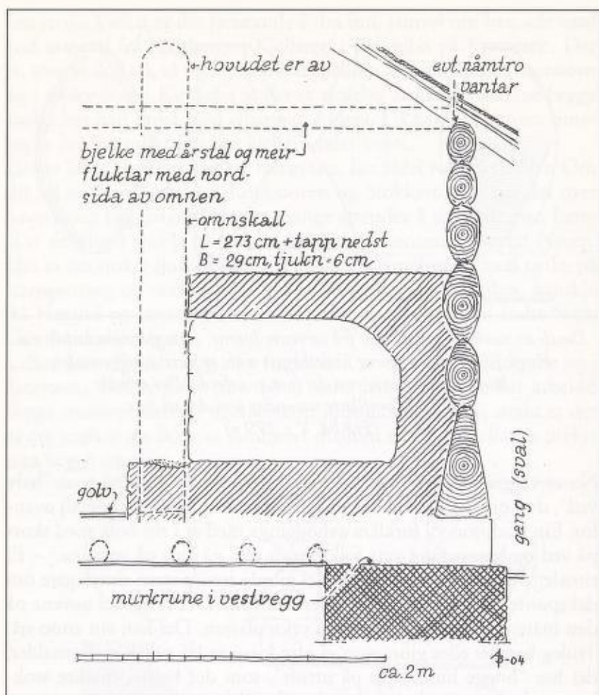
Tenkt snitt gjennom røykonn sett mot sør. (Omskall og omnsbolk er attanfor snittet.)
