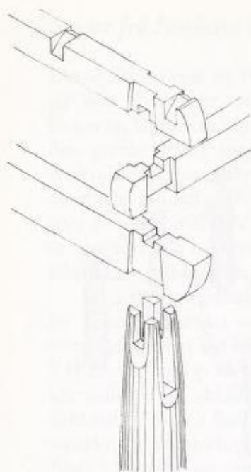
Stav, stavlegjer og bete for samanføying
