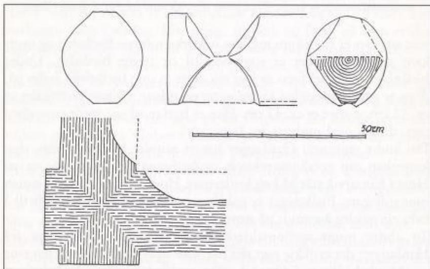
Detalj av novhogg i Roystovan, tilsvarande i Stokkastovan. I plansnittet til venstre viser kor mykje som er avhogge. Men halsen er like heil.
