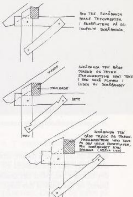
Ulike dømme på innfelling av skråband (sneiband) i stav, bete og stavlegje.
