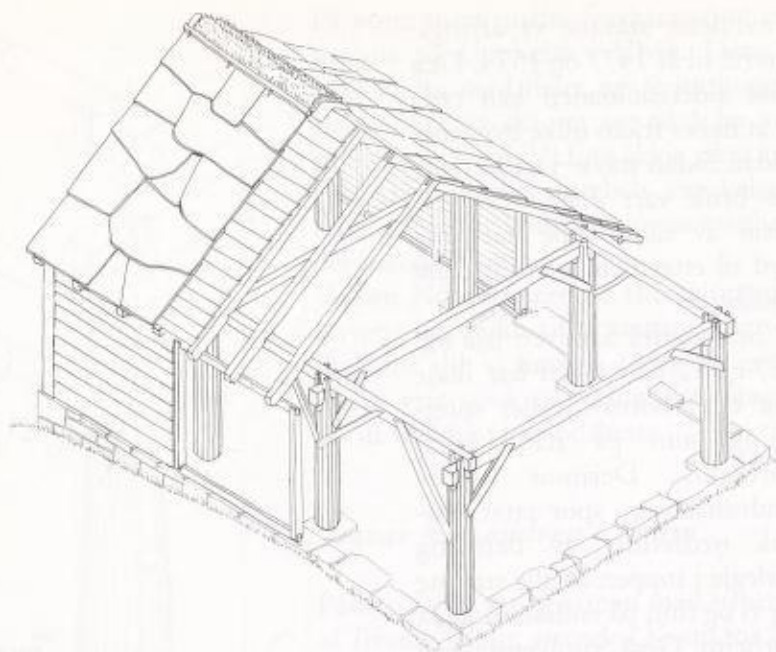
Forsøk på isometrisk snitt av stavløe på Sandven i Kvam
