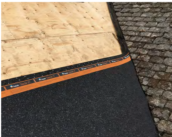
Figur 29. Takpapp rullas ut på det nya underlagstaket av plywood. Foto: Emil Engqvist.
