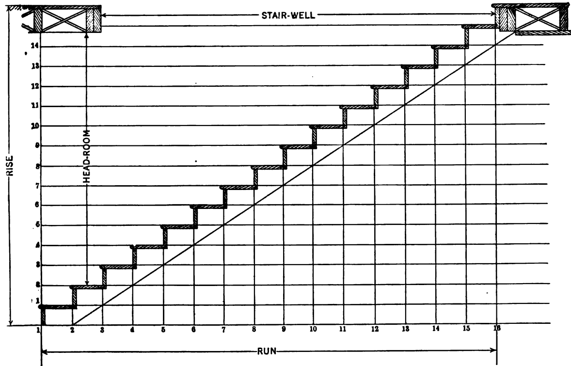
FIG. 52.—Stair Arrangement.
