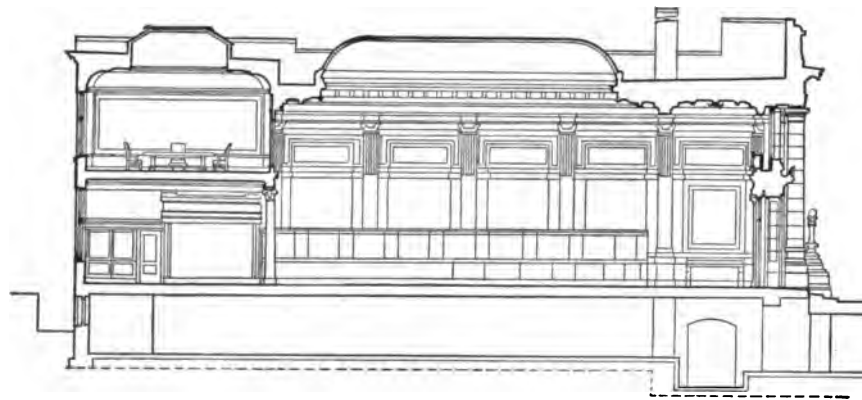
(d) Longitudinal Section on Line X-X.
