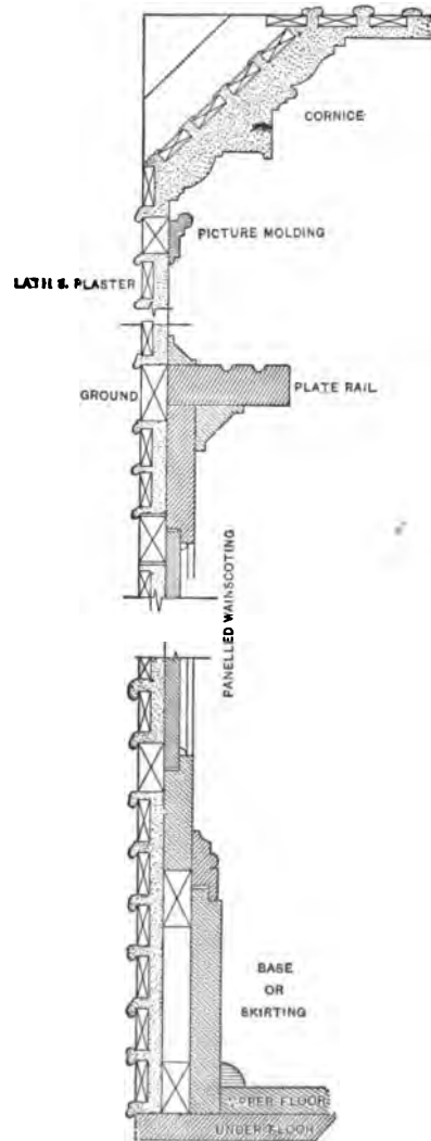
FIG. 48.—Interior Trim.
